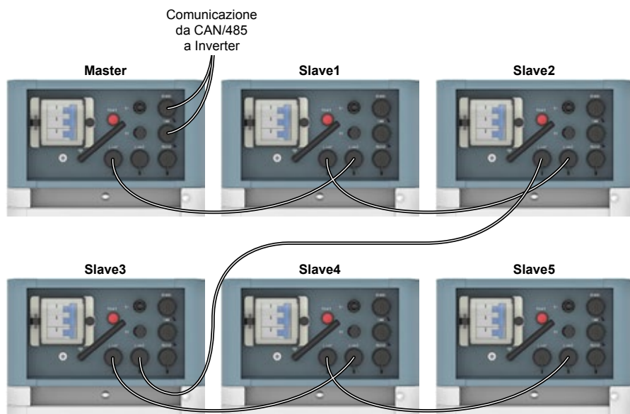
Fig. 3.13 - Schema di collegamento Master/Slave
