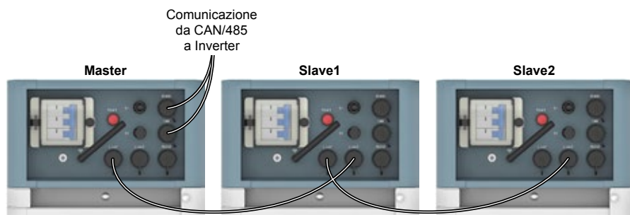
Fig. 3.12 - Schema di collegamento Master/Slave
