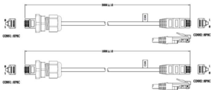
Fig. 3.8 - Cavi di comunicazione
