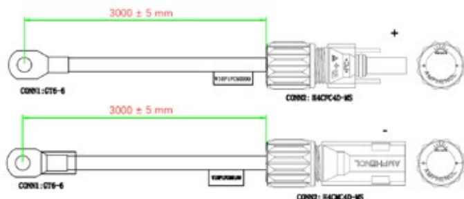
Fig. 3.7 - Cavi di alimentazione
