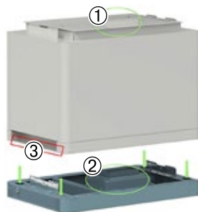
Fig. 4.4 - Il modulo batteria e la base vanno impilati
