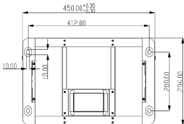
Fig. 3.2 - Fori della base del supporto della batteria
