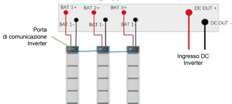
Fig. 3.10 - Schema elettrico del sistema a tre stringhe
