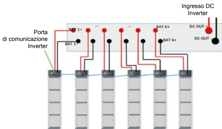
Fig. 3.11 - Schema elettrico del sistema a sei stringhe
