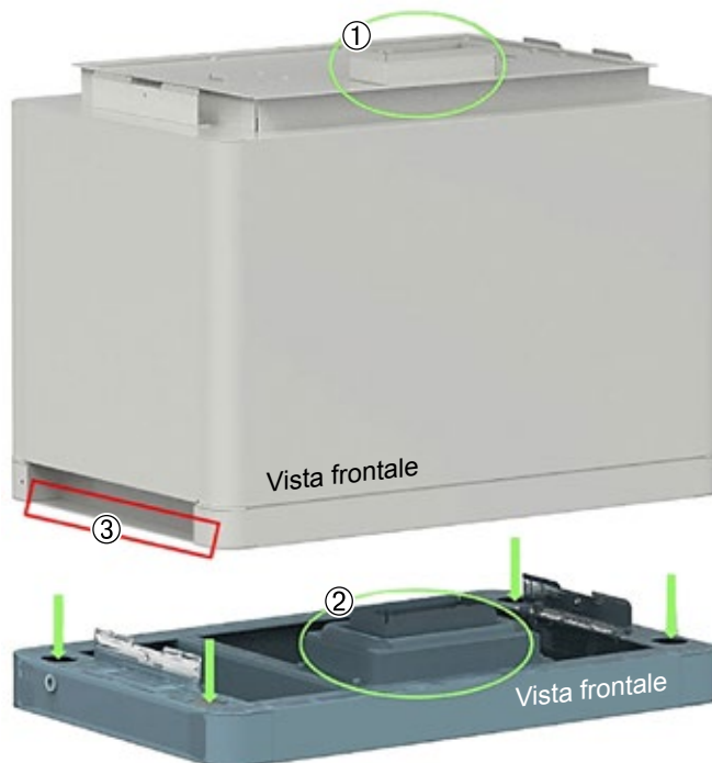
Fig. 3.3 - Il modulo batteria e la base vanno impilati
